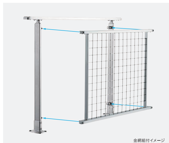
金網組付イメージ
