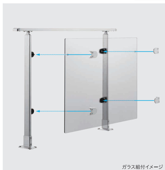
ガラス組付イメージ
