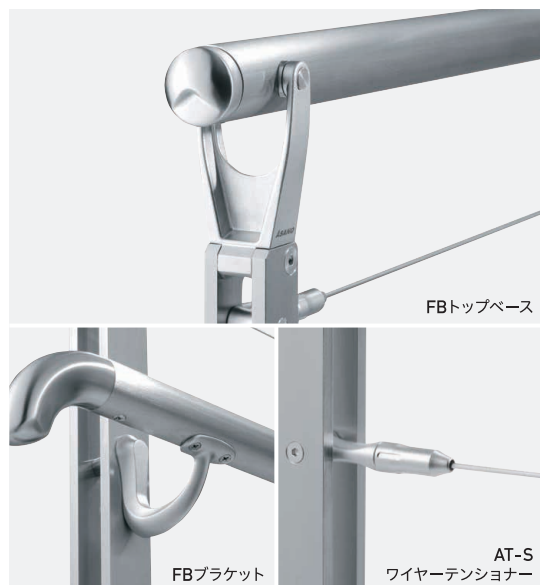
FBブラケット
