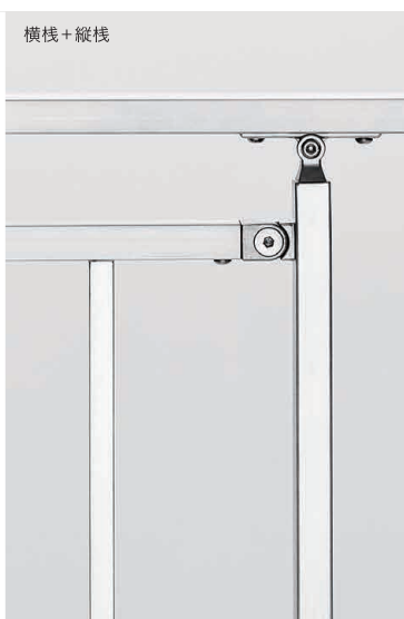
横縦棧組付イメージ
