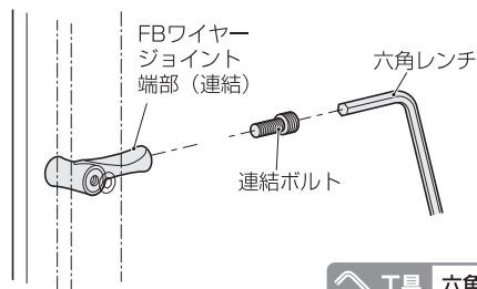
工具 六角レンチ (6mm)
