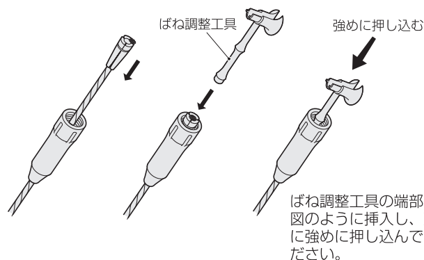
ばね調整工具
