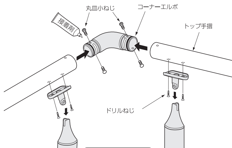
3次元外コーナー
