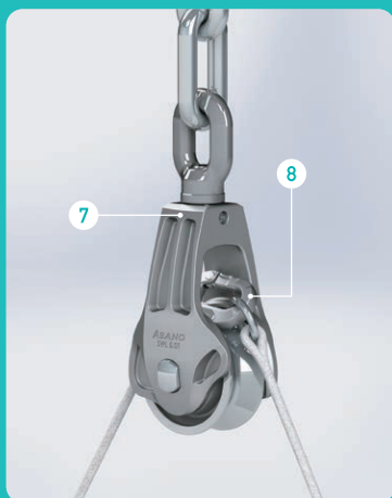
⑦ 強力吊ローラーⅡ型 [P028]
